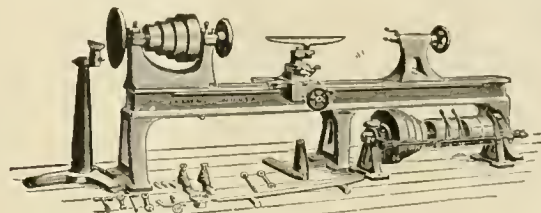
J. A. FAY & EGAN LATHE.
